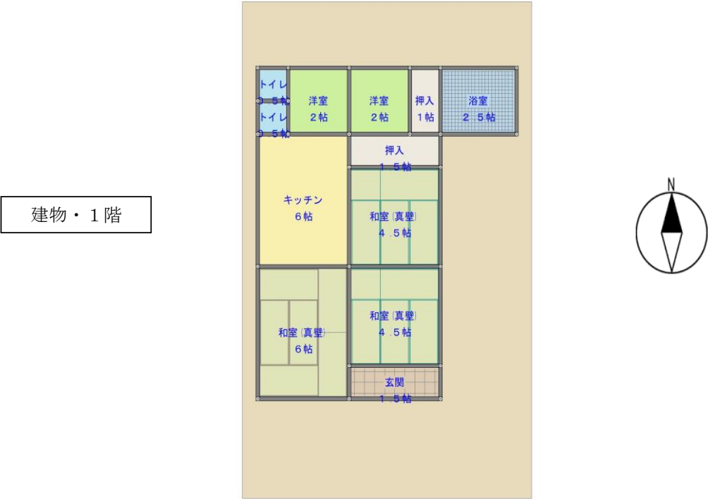
【間取り図】
