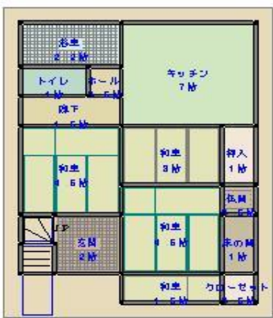
建物・1階
